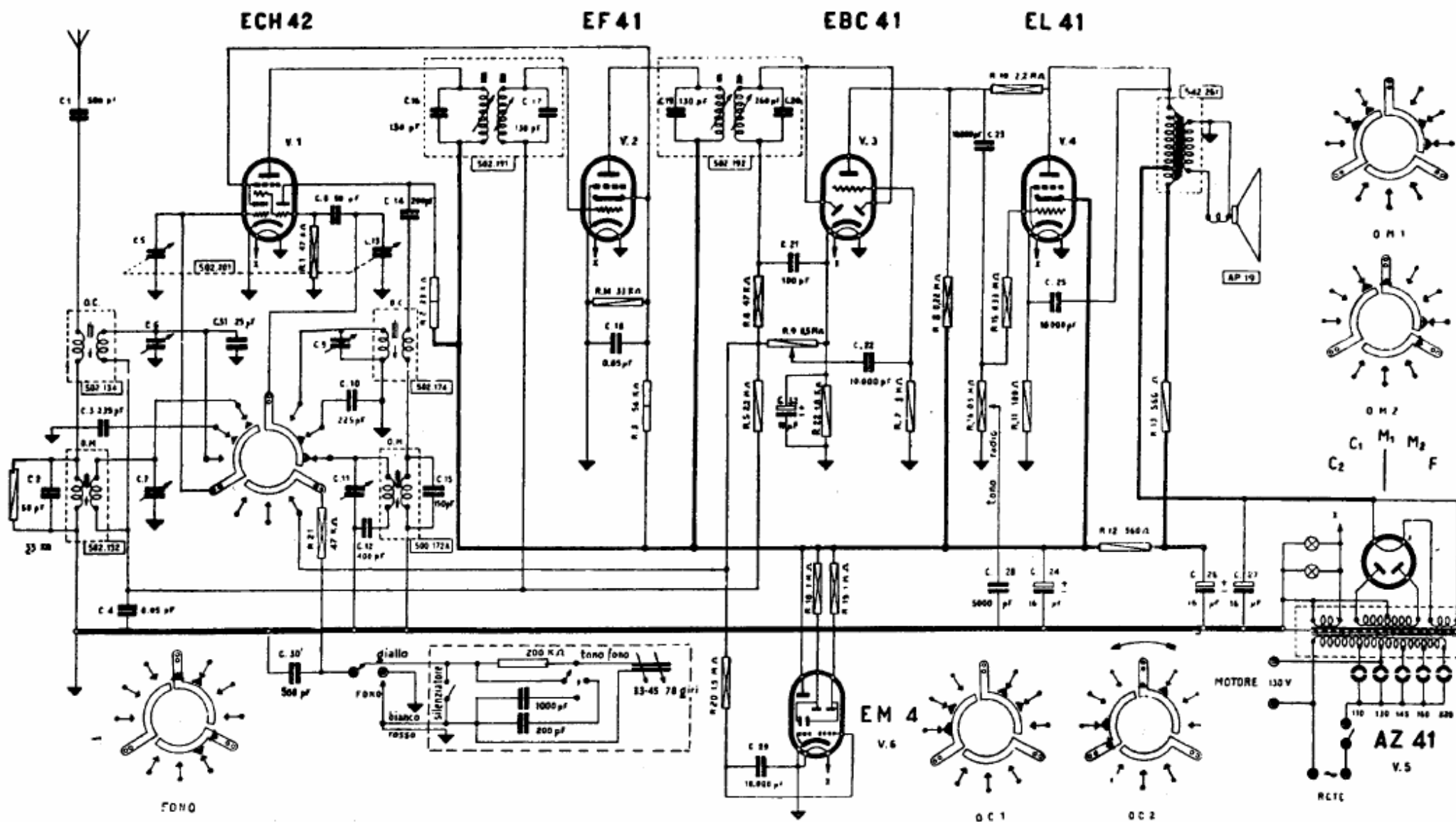
VOCE DEL PADRONE - Mod. Marconi 1543. Radiogrammofono da tavolo. Quattro gamme d'onda: OM1: 430-570 m; OM2: 187-440 m; OC1: 38,5-52 m; OC2: 18-38,5 m. Complesso giradischi a tre velocità, rivelatore con due puntine commutabili per dischi normali a 78 giri e microscolco a 33 e 45 giri. Potenza d'uscita 4 watt. Media frequenza 465 kc.
